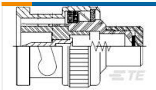
TE 零件编号1-1337523-0 BNC Plg Term 50Ohm Nickel Pltd
